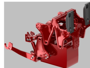
rear_accessories
